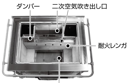
燃焼室アクセスプレート ドミノ8は2枚、ドミノ6は1枚
